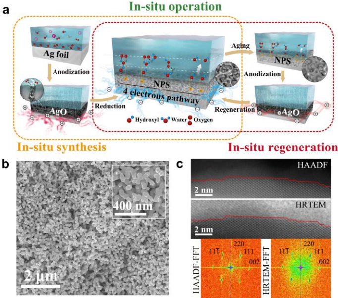
图 1 原理图
